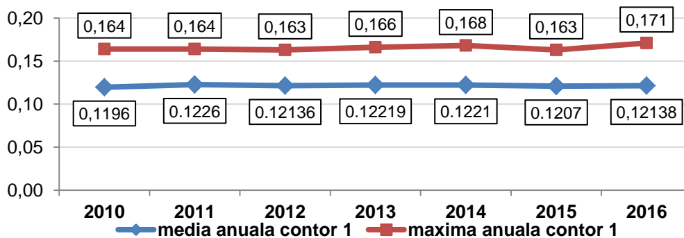
Figura IX.1.1.3. Variația mediilor și maximelor anuale ale debitului dozei gama la contorul 1 al stației automate Bistrița
