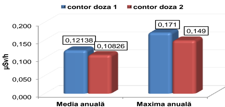
Figura IX.1.1.2. Valorile medii și maxime anuale înregistrate de cele două contoare ( \mu\text{Sv/h} ) stația Bistrița, anul 2016
