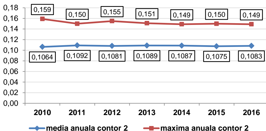
Figura IX.1.1.4. Variația mediilor și maximelor anuale ale debitului dozei gama la contorul 2 al stației automate Bistrița
